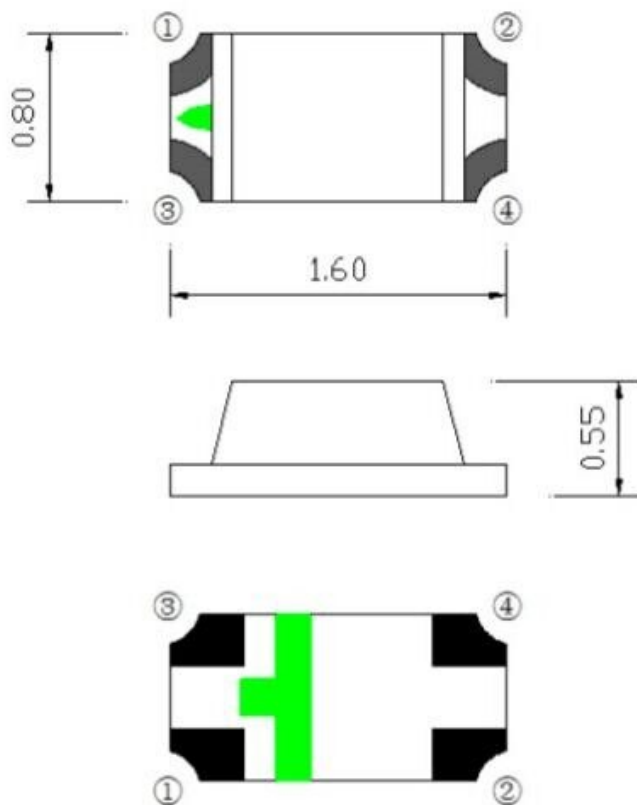
外形尺寸图/ Package Profile
