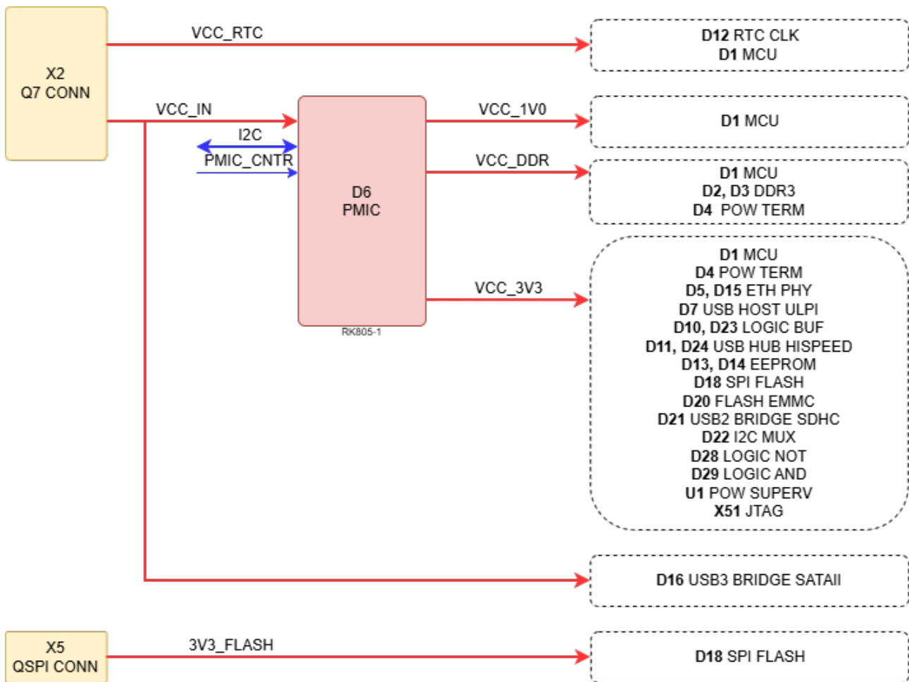
Рисунок 2: Дерево питания
