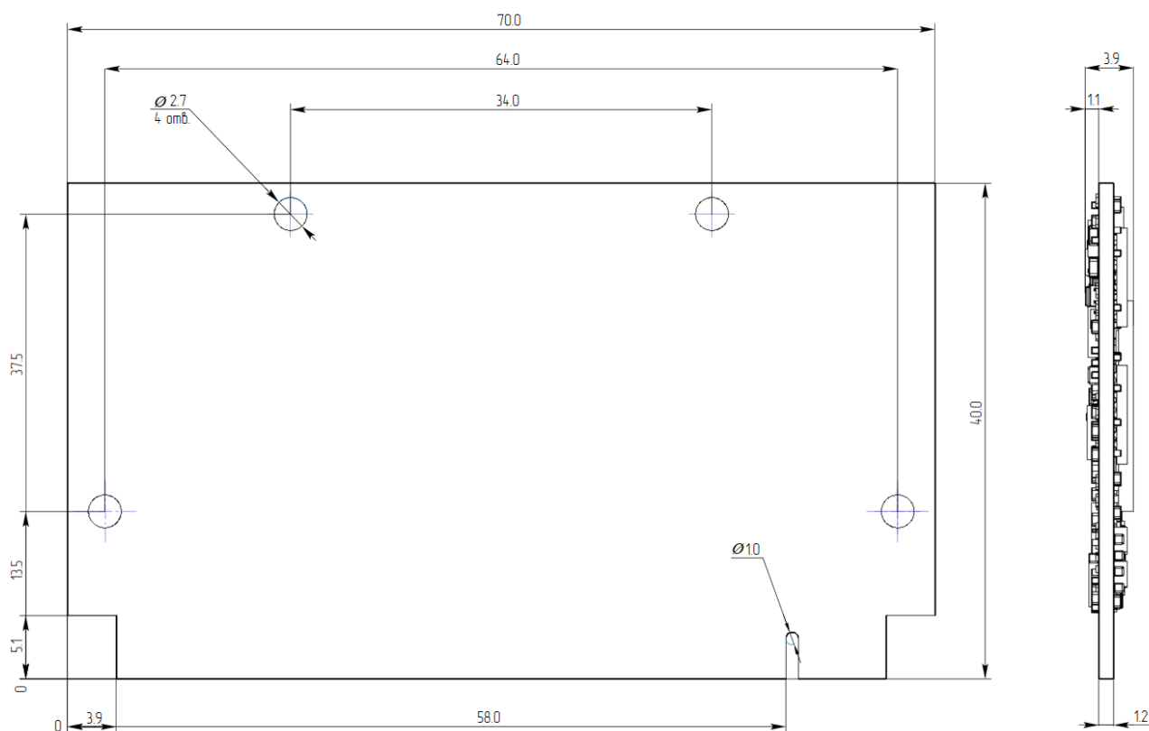
Рисунок 3: Габаритные размеры
