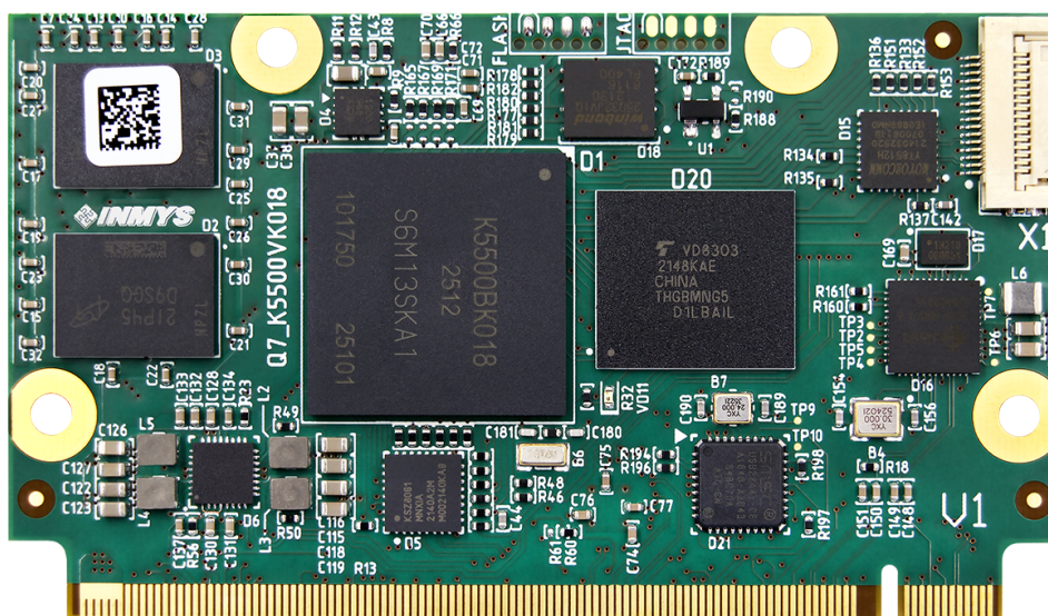
Схемотехника отладочной платы NMS-Q7-EVM-MINI
