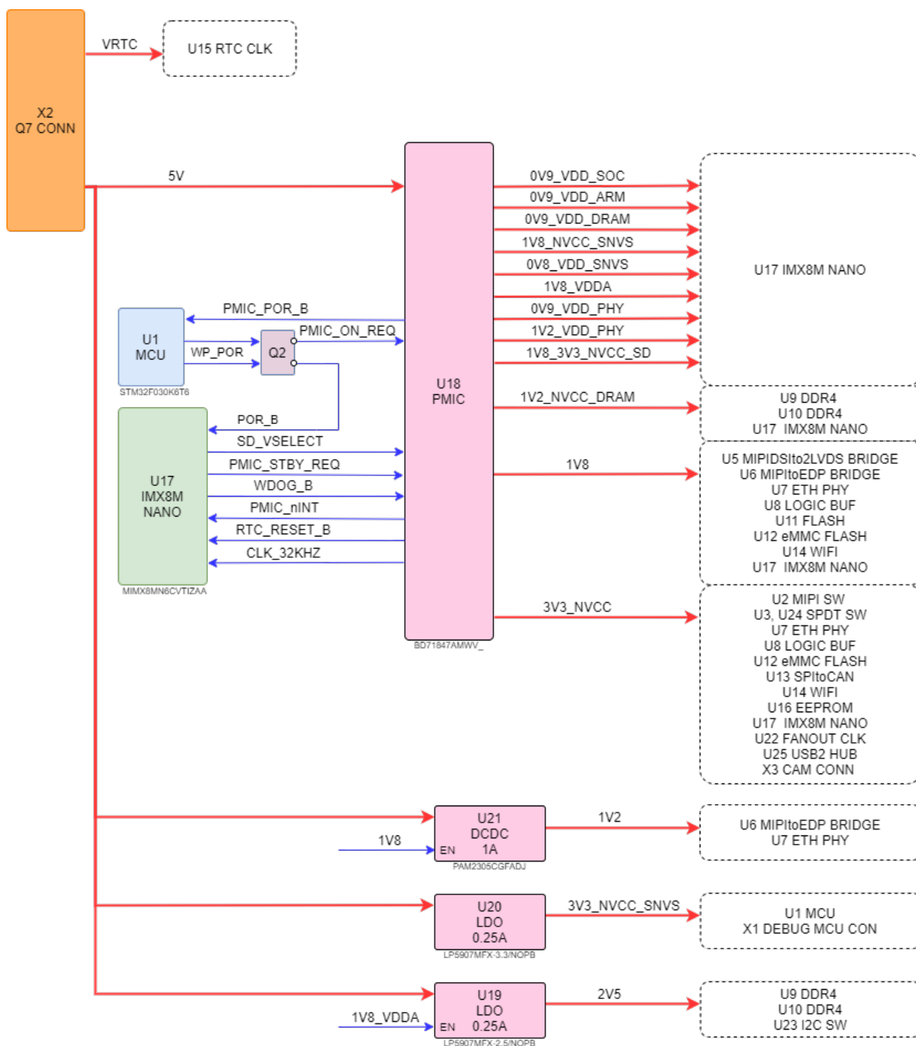
Рисунок 2: Дерево питания
