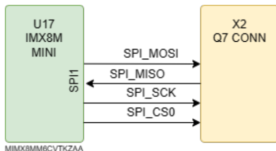
Рисунок 10: Интерфейс SPI
