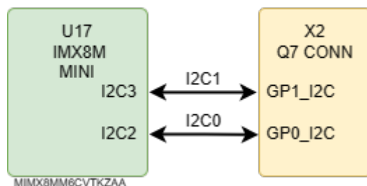
Рисунок 9: I2C интерфейс
