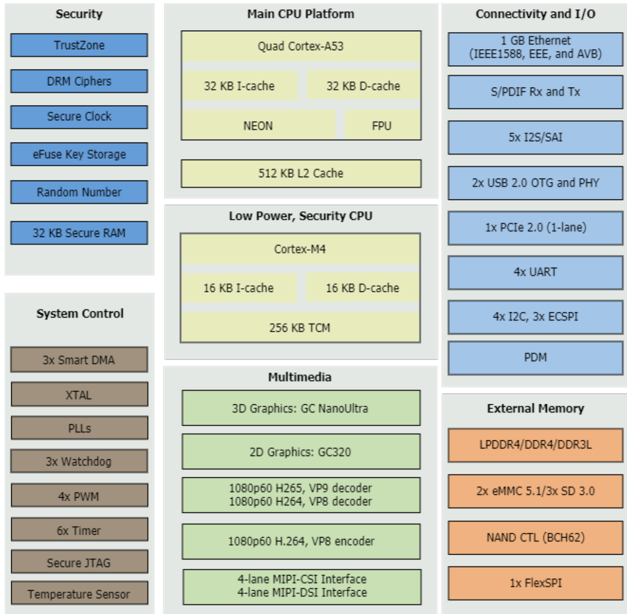
Рисунок 6: Функциональные модули i.MX8M mini
