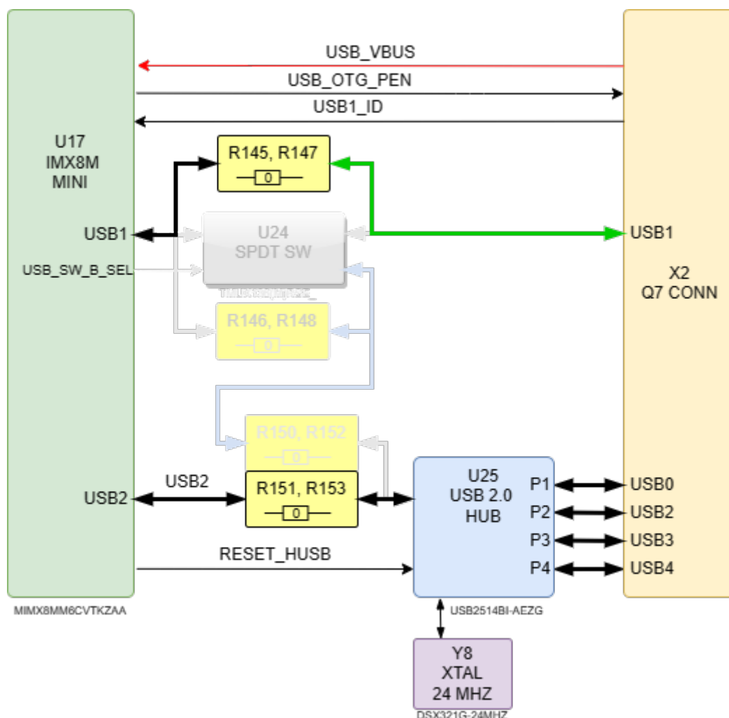
Рисунок 16: Блок-схема PCIe
