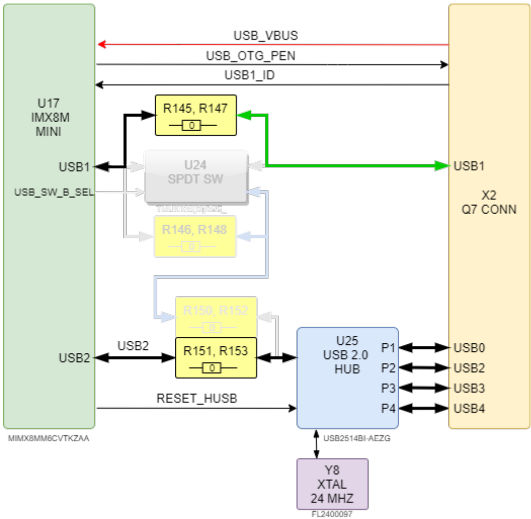
Рисунок 15: Блок-схема USB
