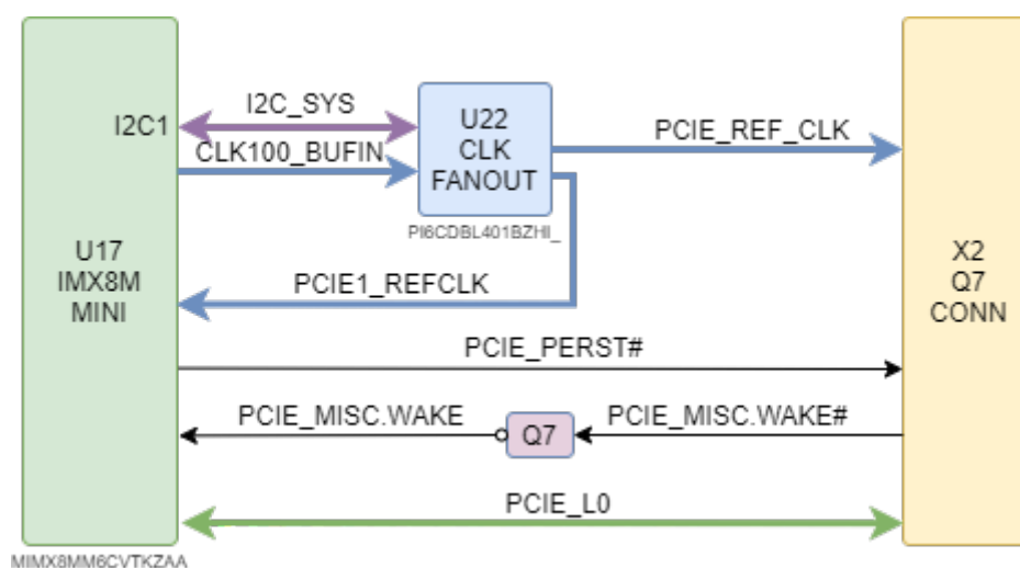
Рисунок 16: Блок-схема PCIe
