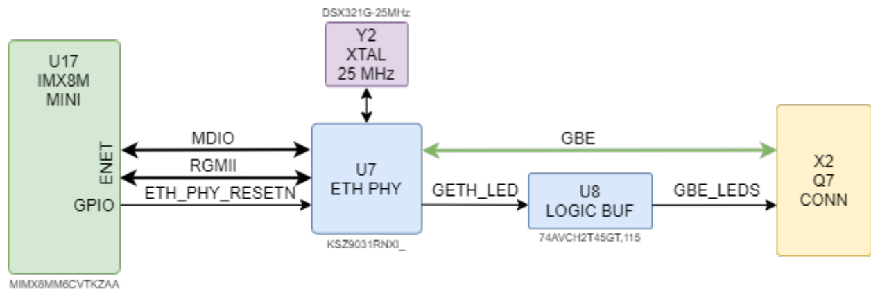
Рисунок 17: Гигабит Ethernet
