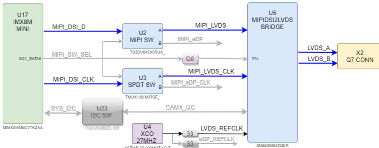
Рисунок 13: Интерфейс LVDS
