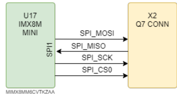
Рисунок 10: Интерфейс SPI
