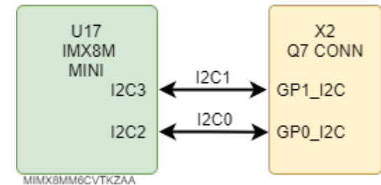
Рисунок 9: I2C интерфейс
