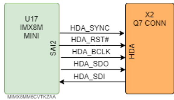
Рисунок 12: Аудио интерфейс
