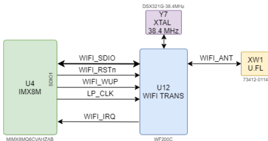
Рисунок 8: Wi-Fi связи
