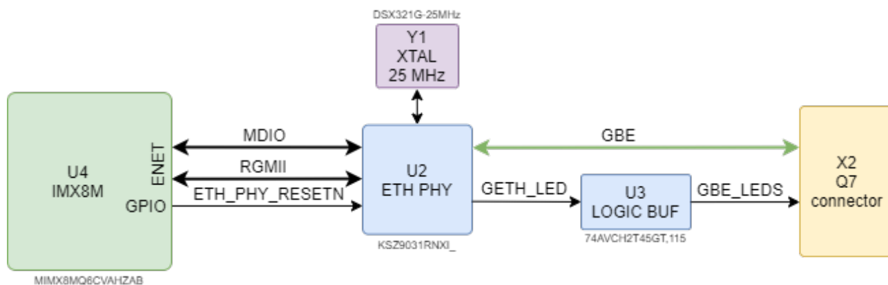
Рисунок 13: Гигабит Ethernet
