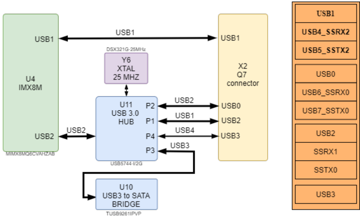
Рисунок 10: Блок-схема USB
