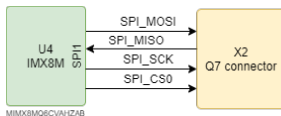
Рисунок 17: Интерфейс SPI
