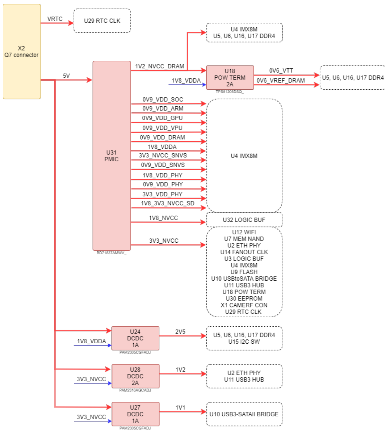
Рисунок 2: Дерево питания
