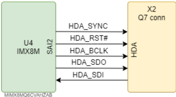
Рисунок 20: Аудио интерфейс
