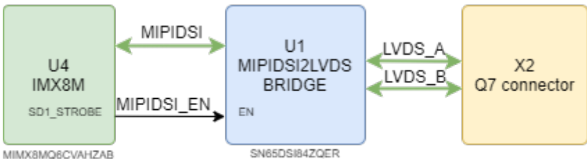
Рисунок 21: Интерфейс LVDS
