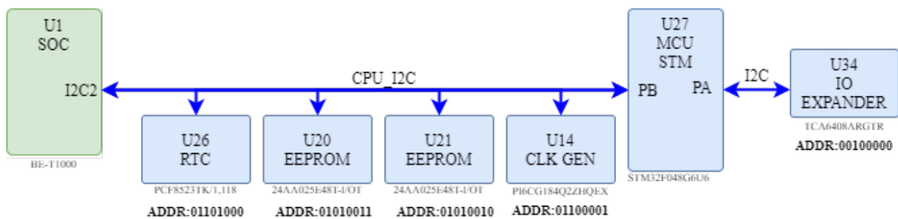
Рисунок 8: I2C интерфейс
