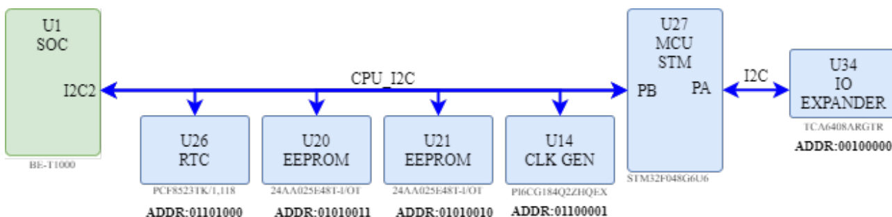
Рисунок 8: I2C interface
