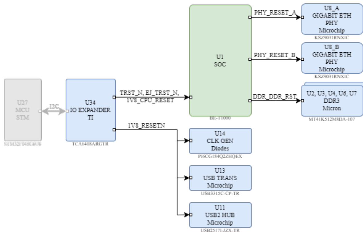
Рисунок 9: Reset signals
