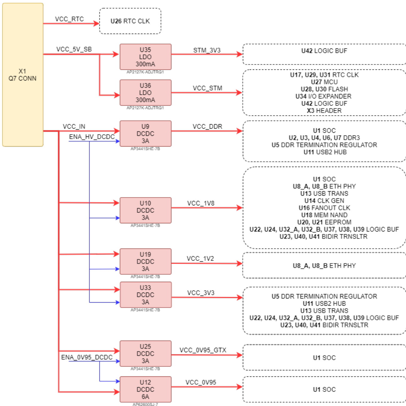
Рисунок 2: Power tree
