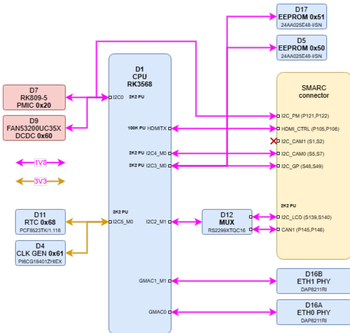
Рисунок 6: I2C интерфейс
