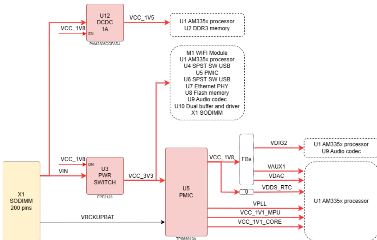
Рисунок 2: Дерево питания
