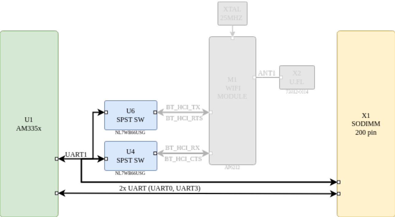
Рисунок 7: UART интерфейс
