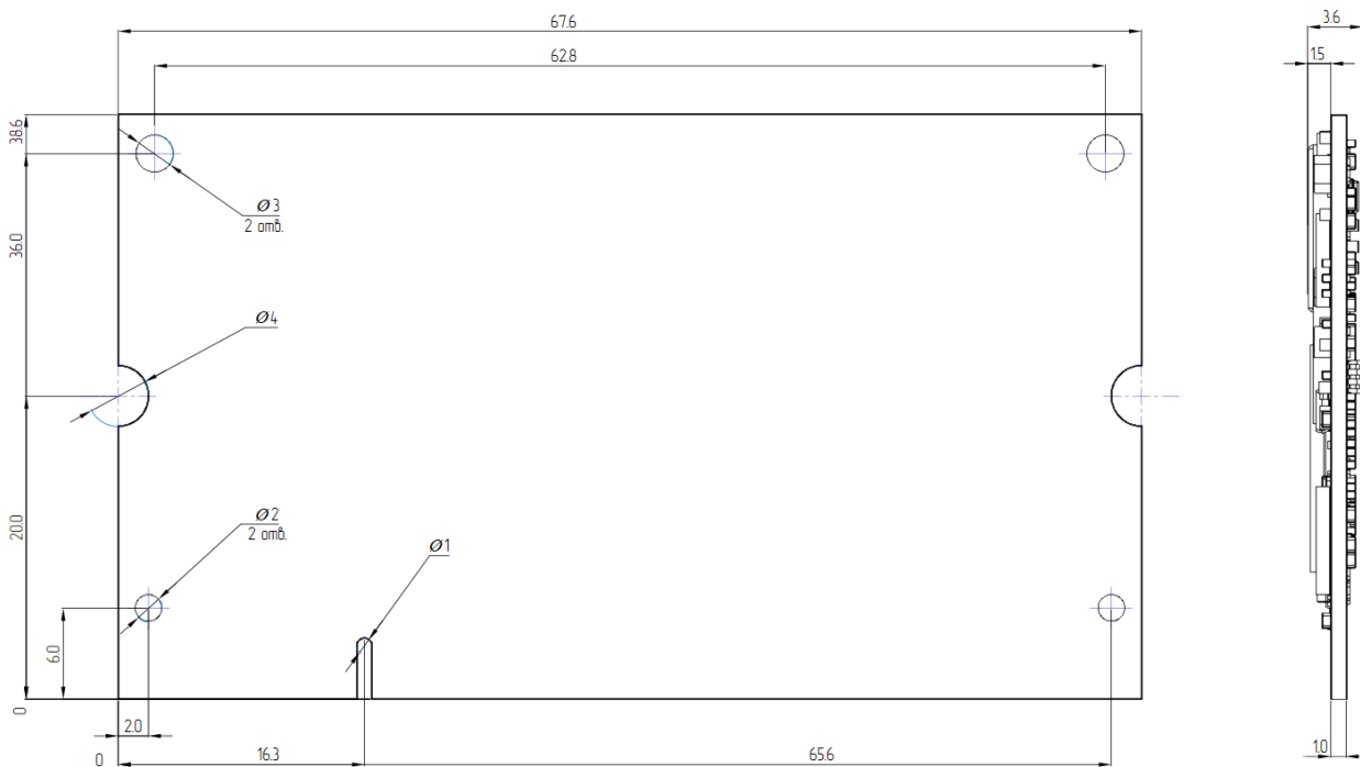
Рисунок 3: Габаритные размеры
