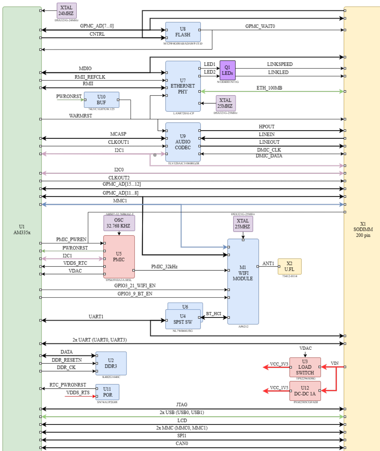
Рисунок 1: Структурная схема модуля
