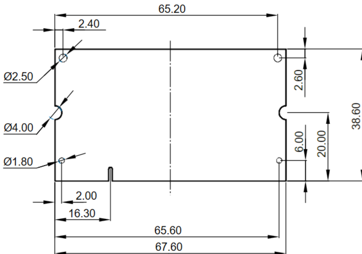
Рисунок 3: Габаритные размеры
