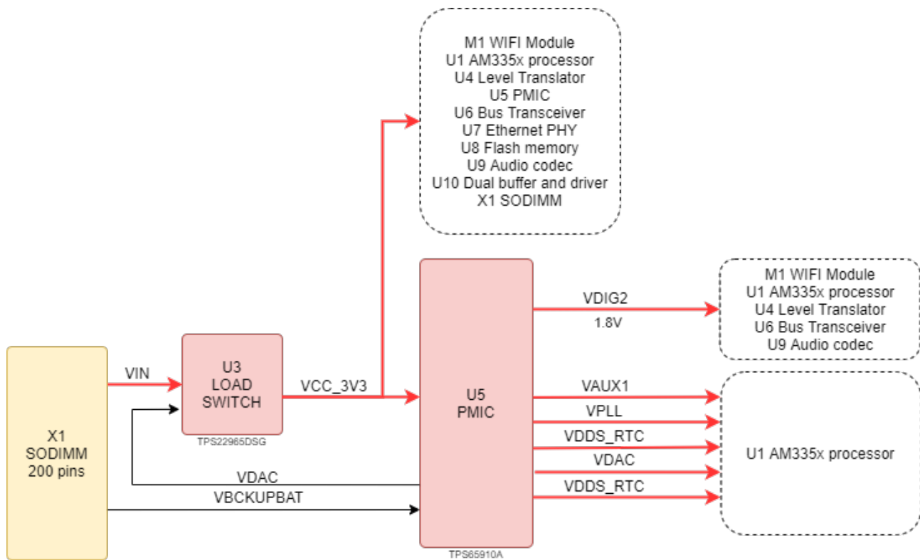
Рисунок 2: Дерево питания
