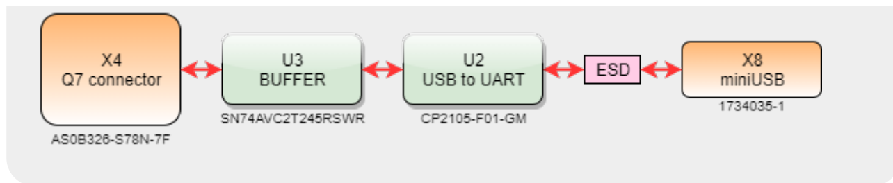
Рисунок 8: Отладочная консоль USB
