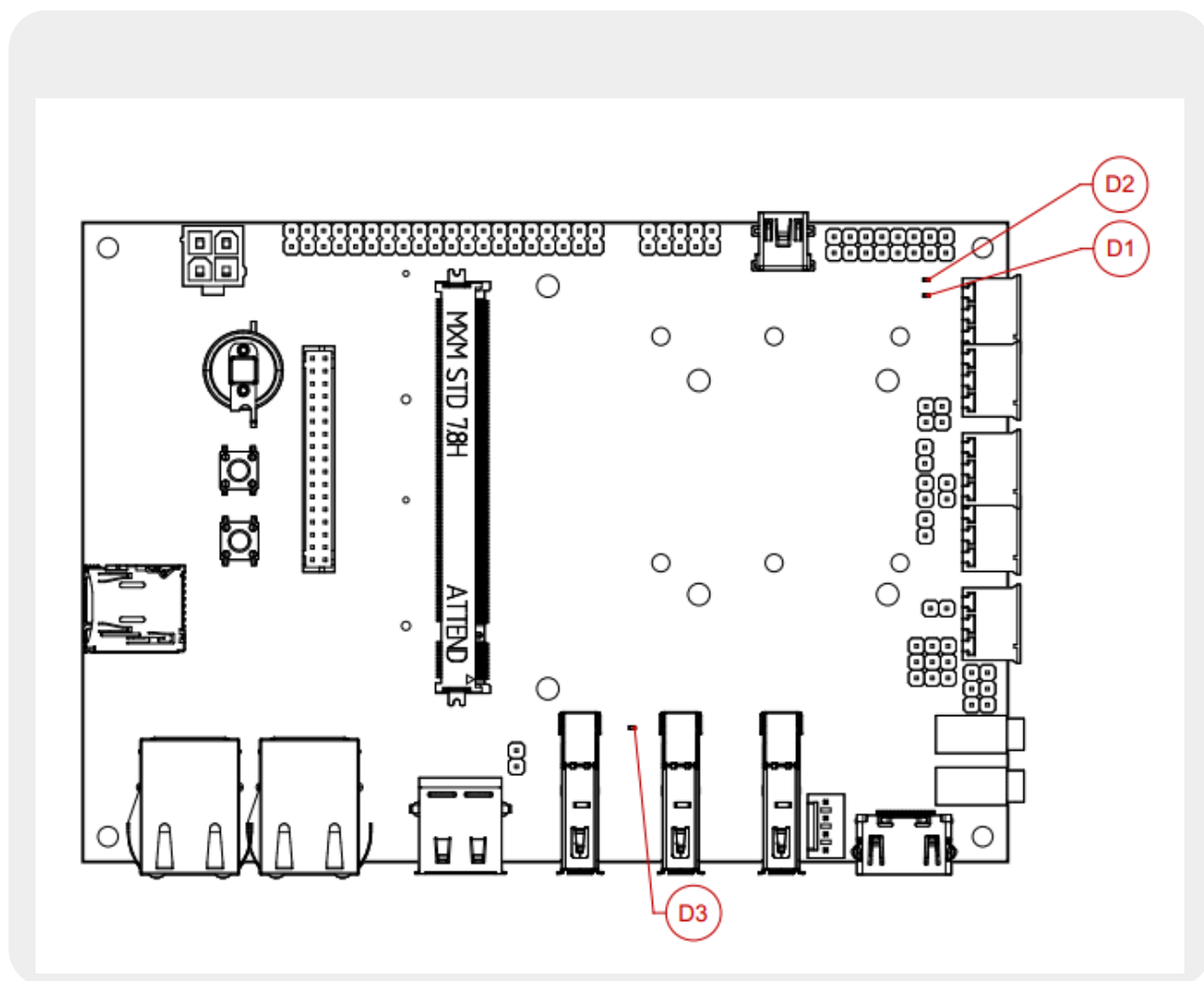
Рисунок 16: Расположение светодиодов на плате nms-q7-evm
