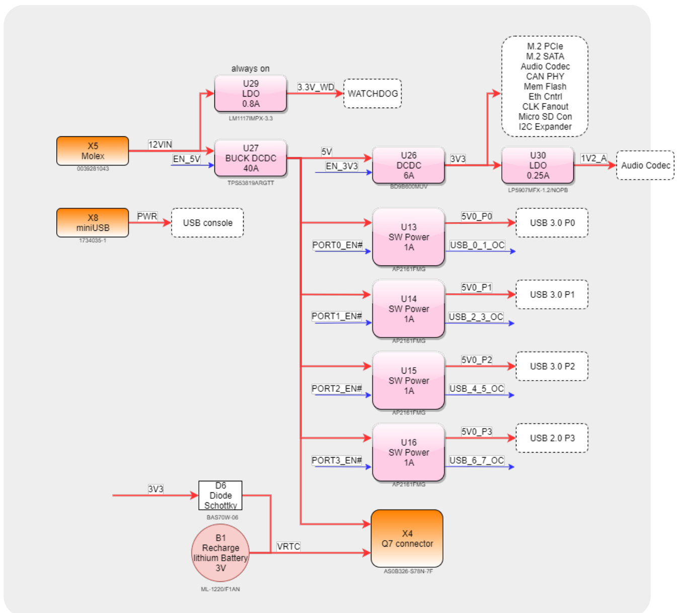
Рисунок 2: Дерево питания
