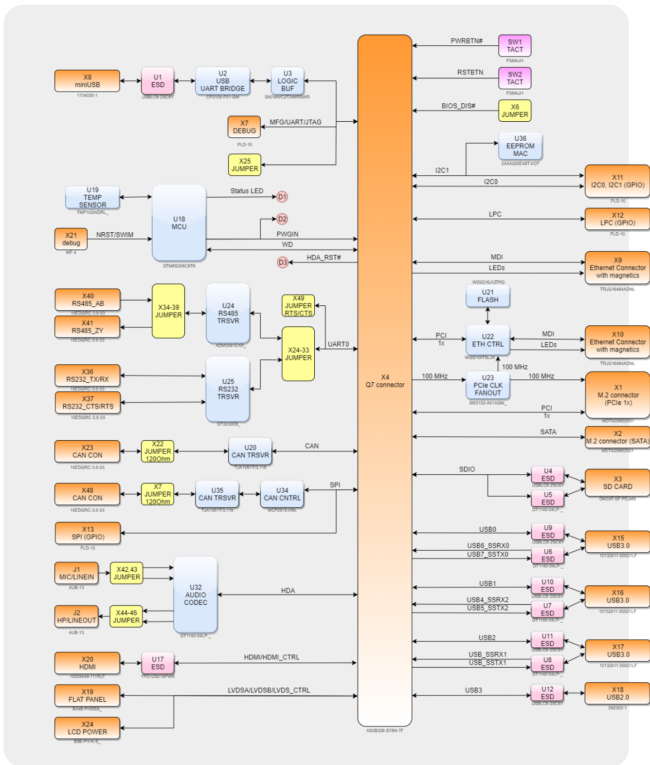
Рисунок 1: Блок-схема
