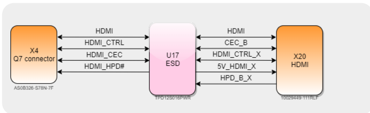
Рисунок 7: Интерфейс HDMI
