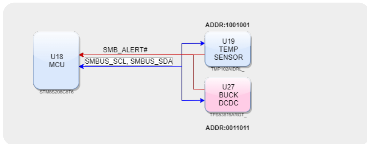
Рисунок 14: Подключение микроконтроллера STM8
