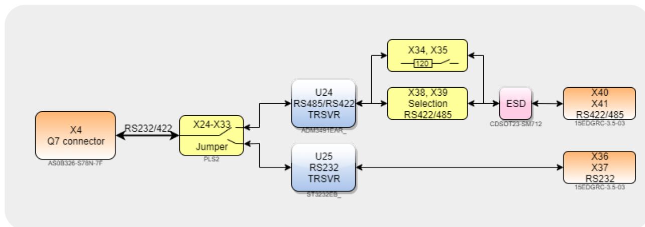
Рисунок 9: Блок-схема Rs232/422/485
