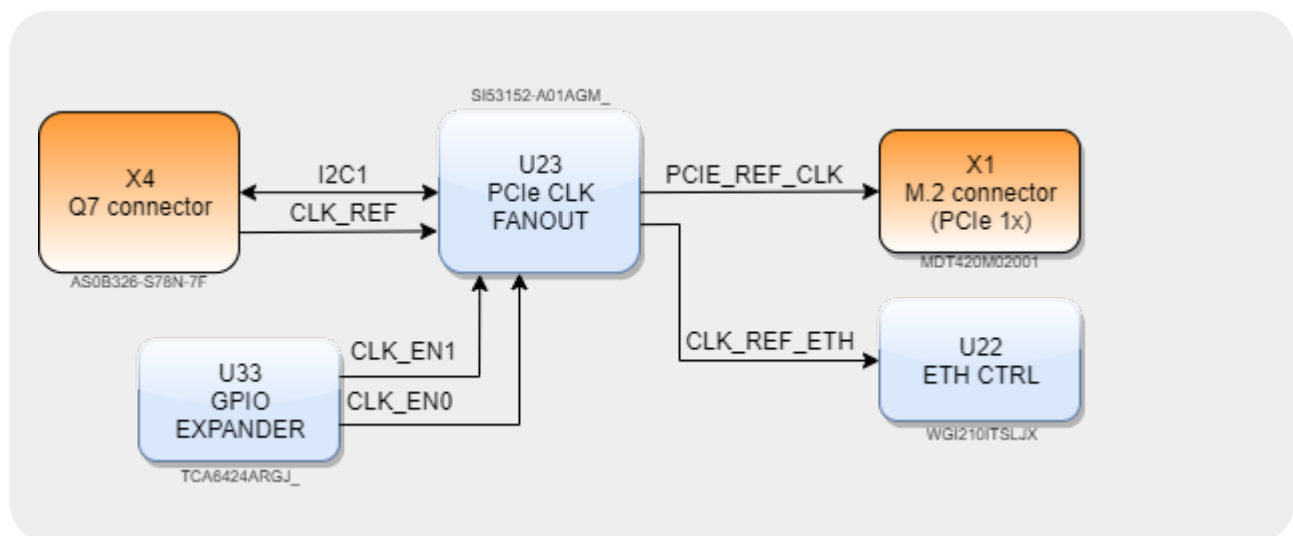
Рисунок 16: Q7Base PCIe clock buffer
