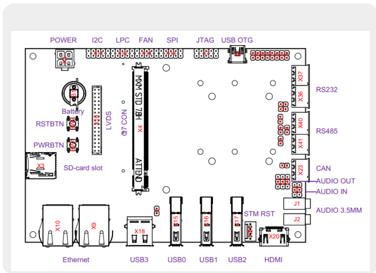
Рисунок 4: Q7Base top components view
