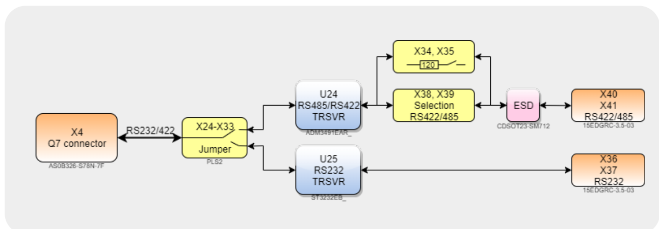
Рисунок 9: Q7Base serial diagram
