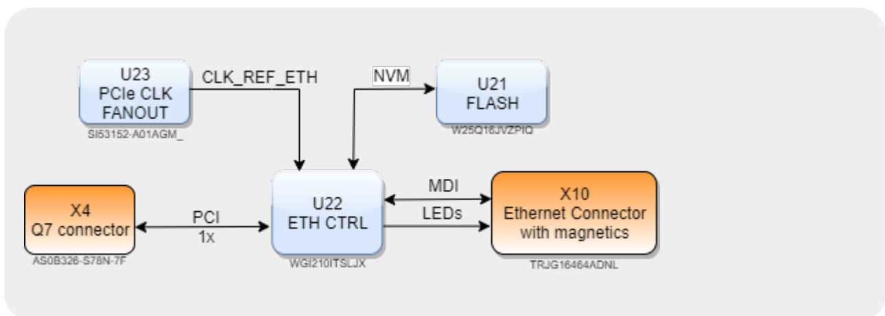
Рисунок 12: Q7Base ethernet diagram
