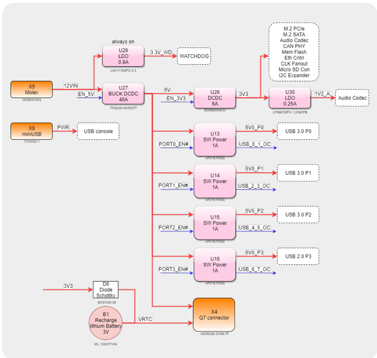
Рисунок 2: Q7Base power tree
