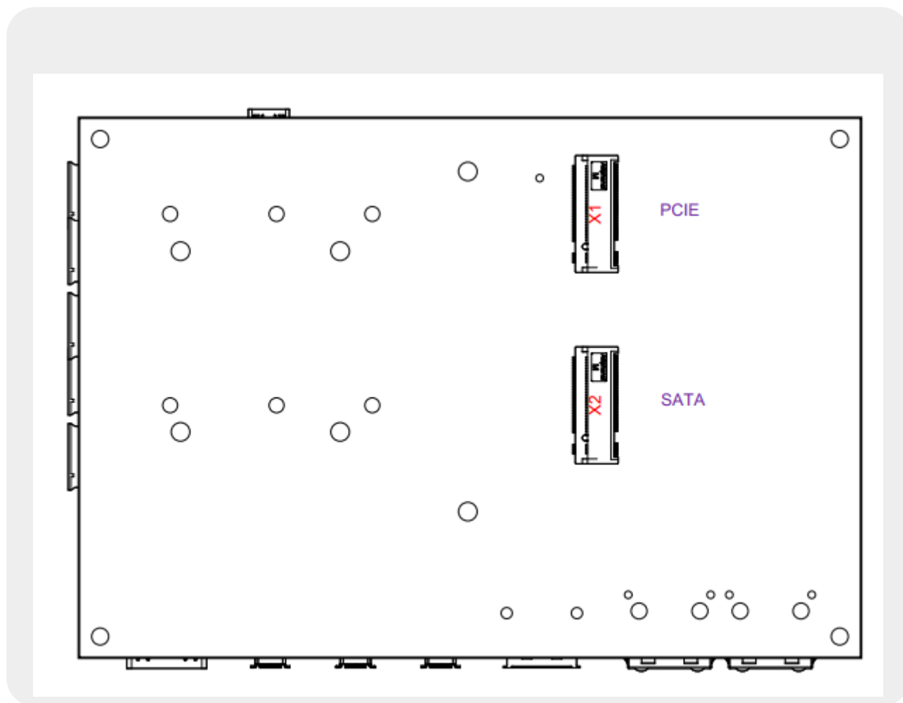
Рисунок 5: Q7Base bot components view
