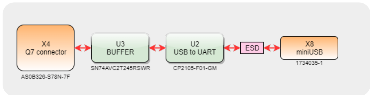
Рисунок 8: Q7Base USB debug console
