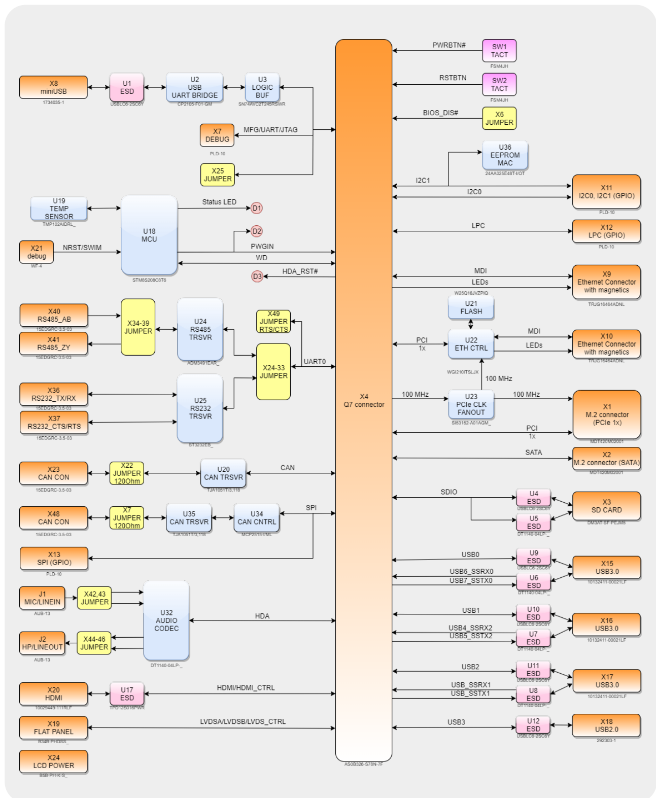
Рисунок 1: Q7Base block diagram
