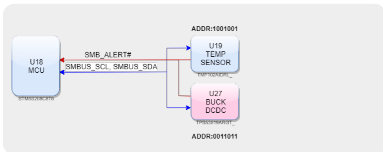
Рисунок 15: Q7Base MCU connections
