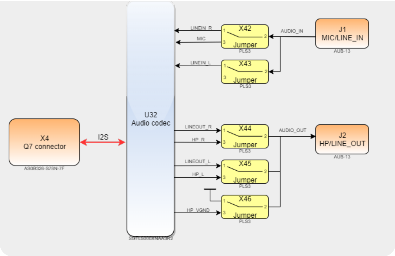
Рисунок 11: Q7Base audio diagram
