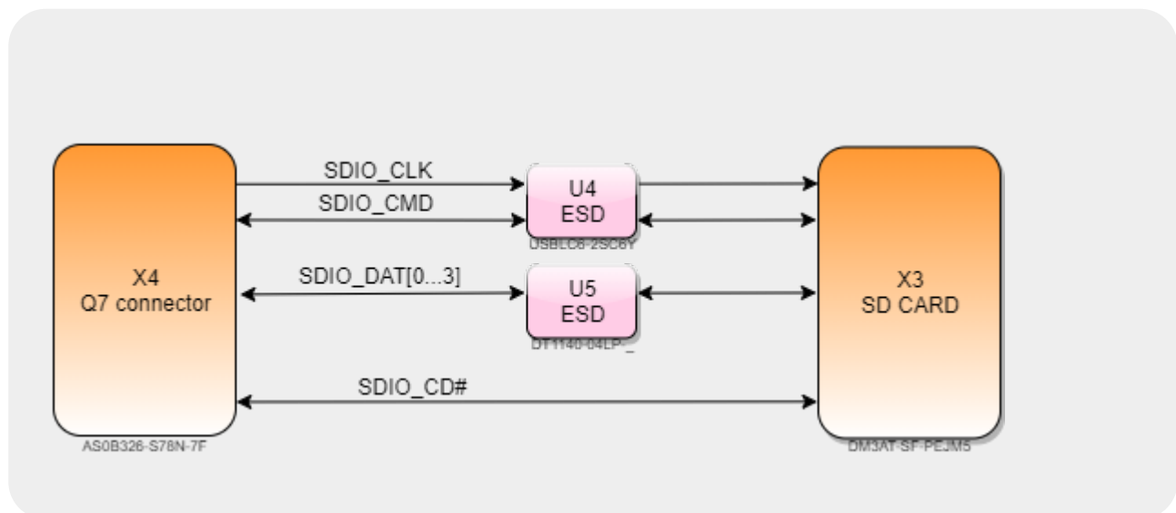
Рисунок 13: Q7Base sdio diagram
