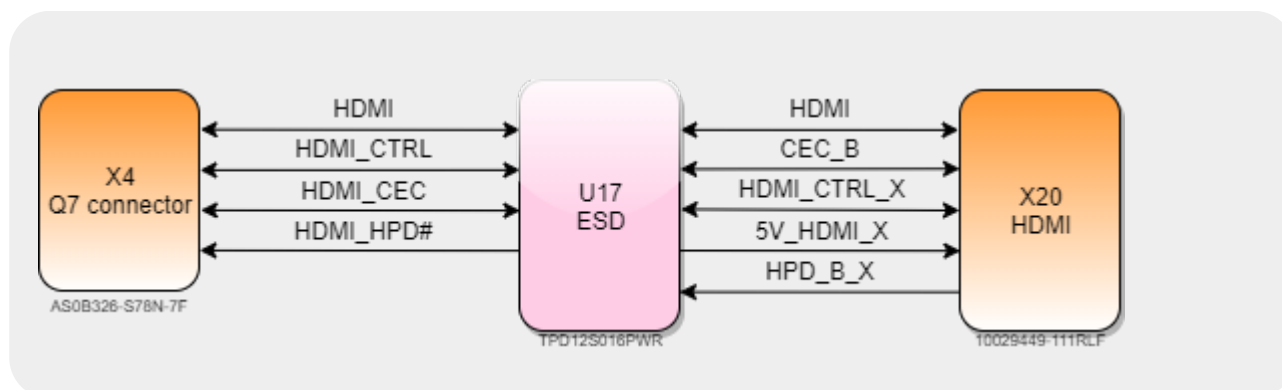
Рисунок 7: HDMI Q7Base
