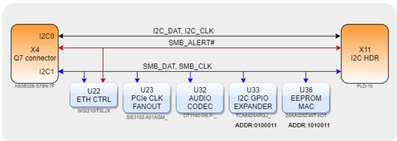
Рисунок 6: I2C Q7Base
