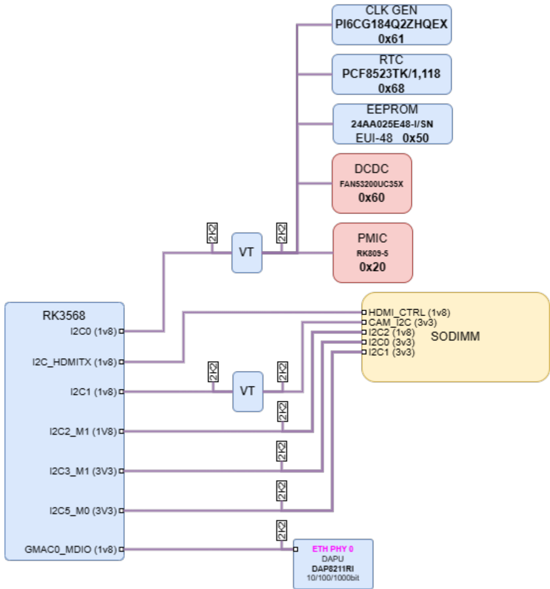
Рисунок 6: I2C интерфейс
