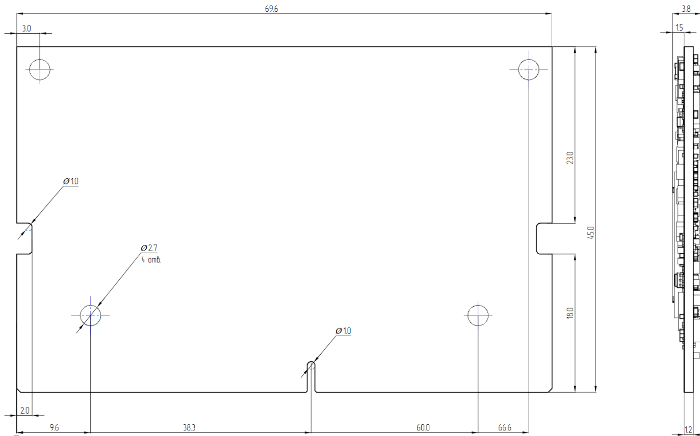
Рисунок 2: Габаритные размеры
