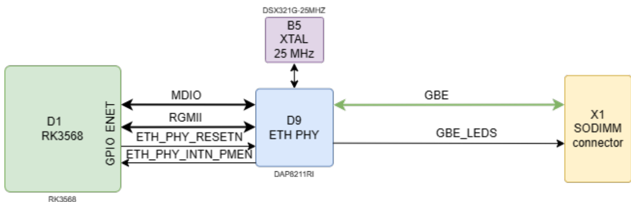
Рисунок 7: Гигабит Ethernet
