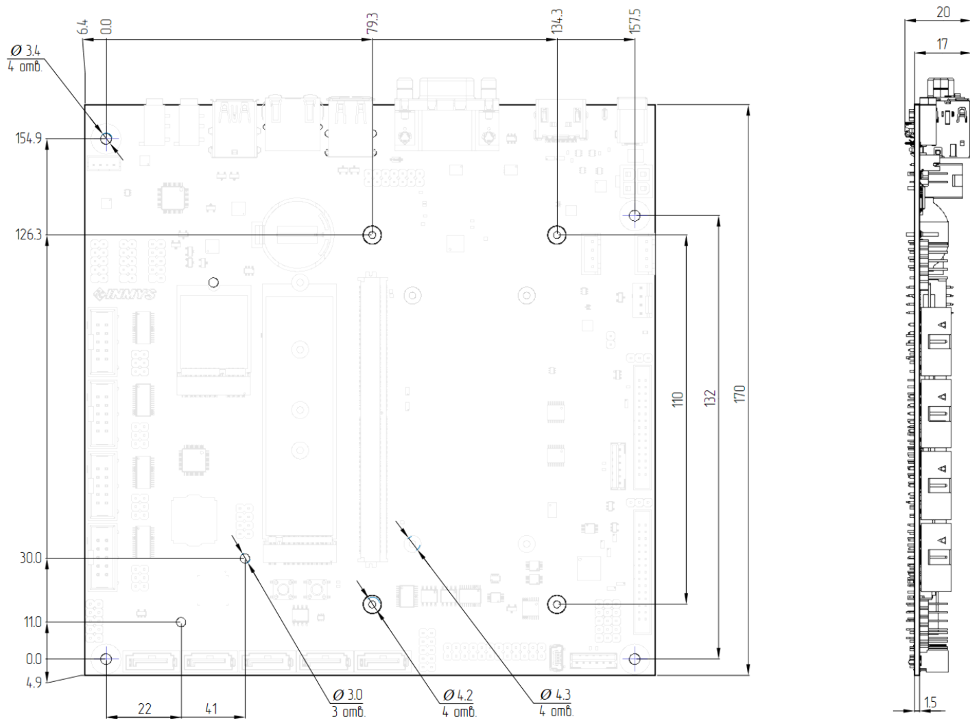
Рисунок 1: Габаритные размеры
