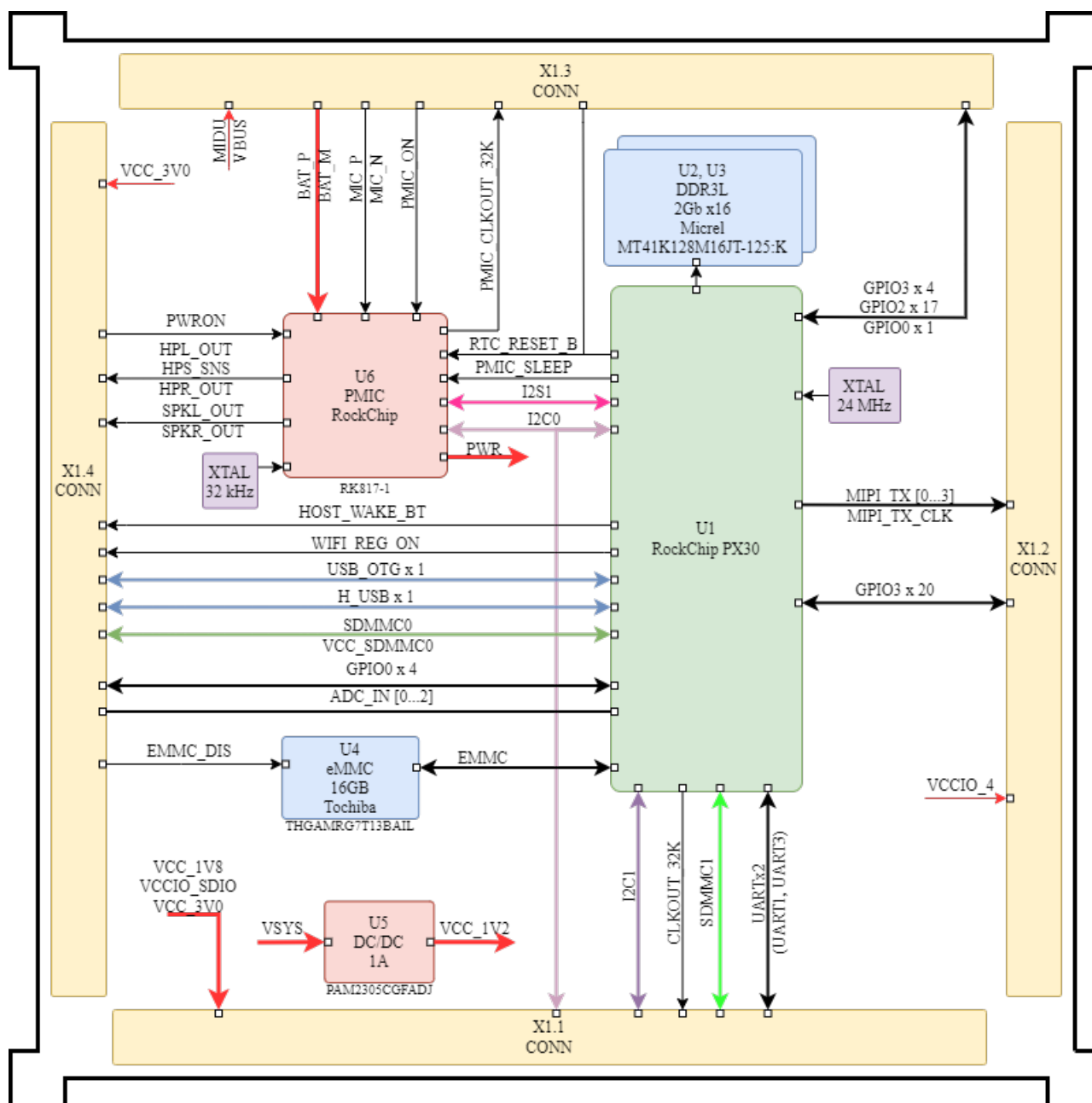
Рисунок 1: Структурная схема модуля
