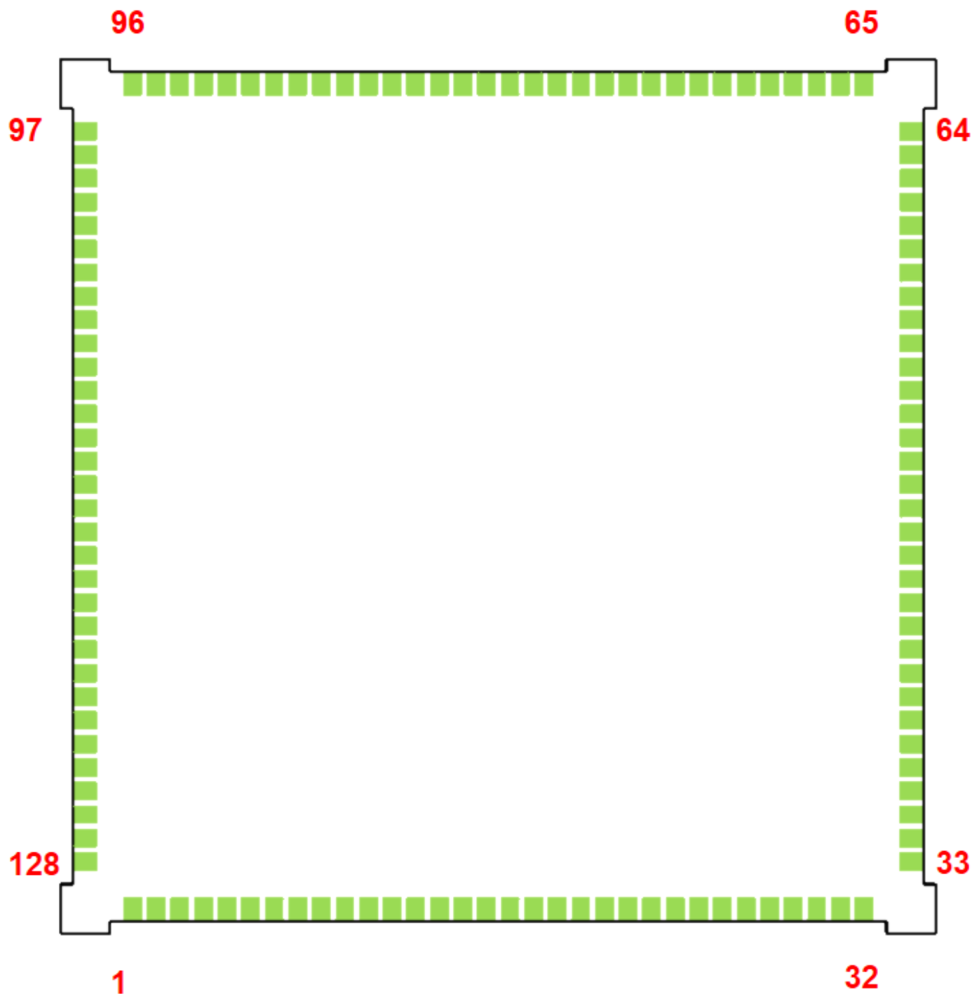
Рисунок 6: Расположение разъемов на плате. Вид сверху
