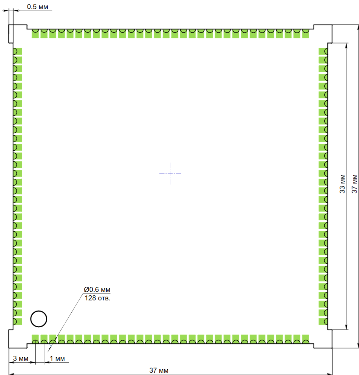
Рисунок 2: Габаритные размеры
