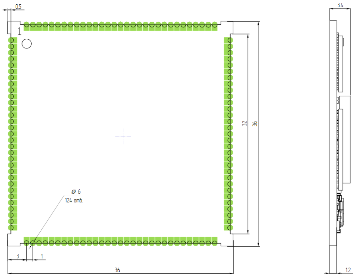
Рисунок 2: Габаритные размеры
