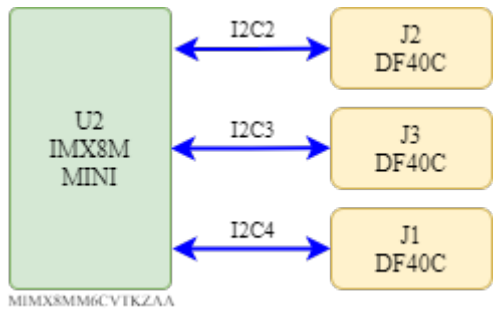
Рисунок 6: I2C интерфейсы
