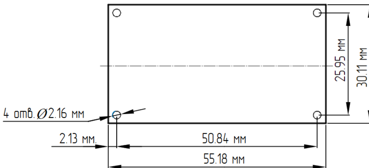
Рисунок 3: Габаритные размеры
