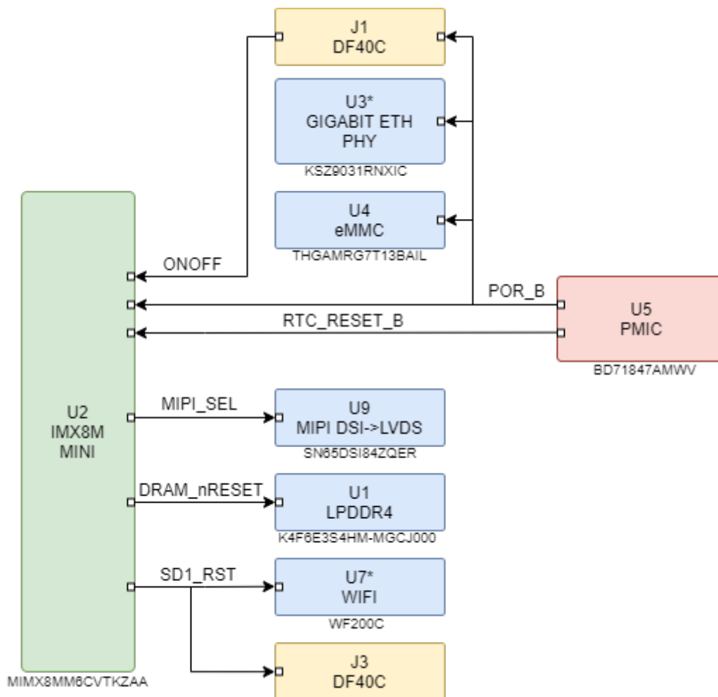
Рисунок 8: Сигналы сброса
