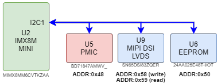
Рисунок 7: I2C1 интерфейс
