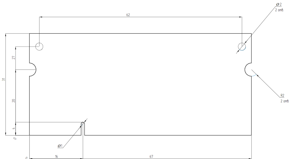
Рисунок 2: Габаритные размеры
