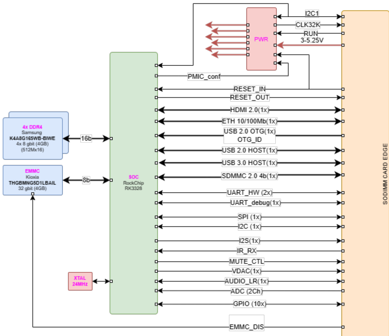
Рисунок 1: Структурная схема модуля
