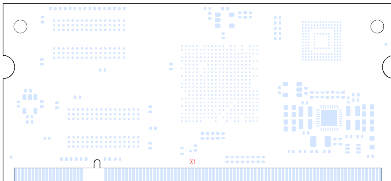
Рисунок 6: Расположение разъемов на плате. Вид сверху
