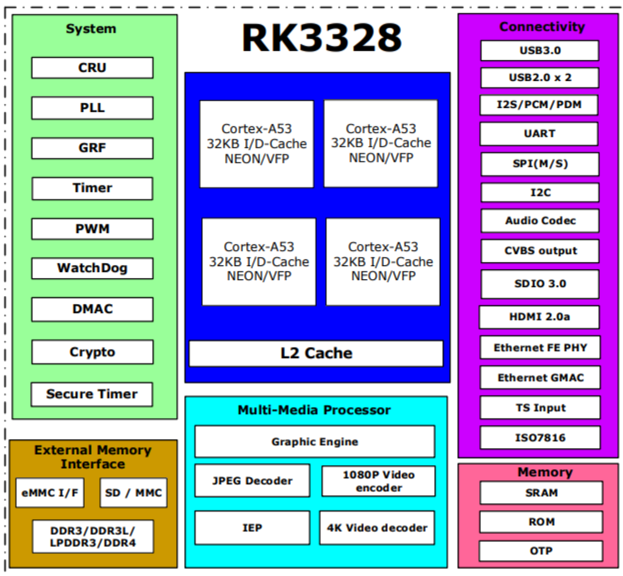
Рисунок 5: Функциональные модули Rockchip RK3328
