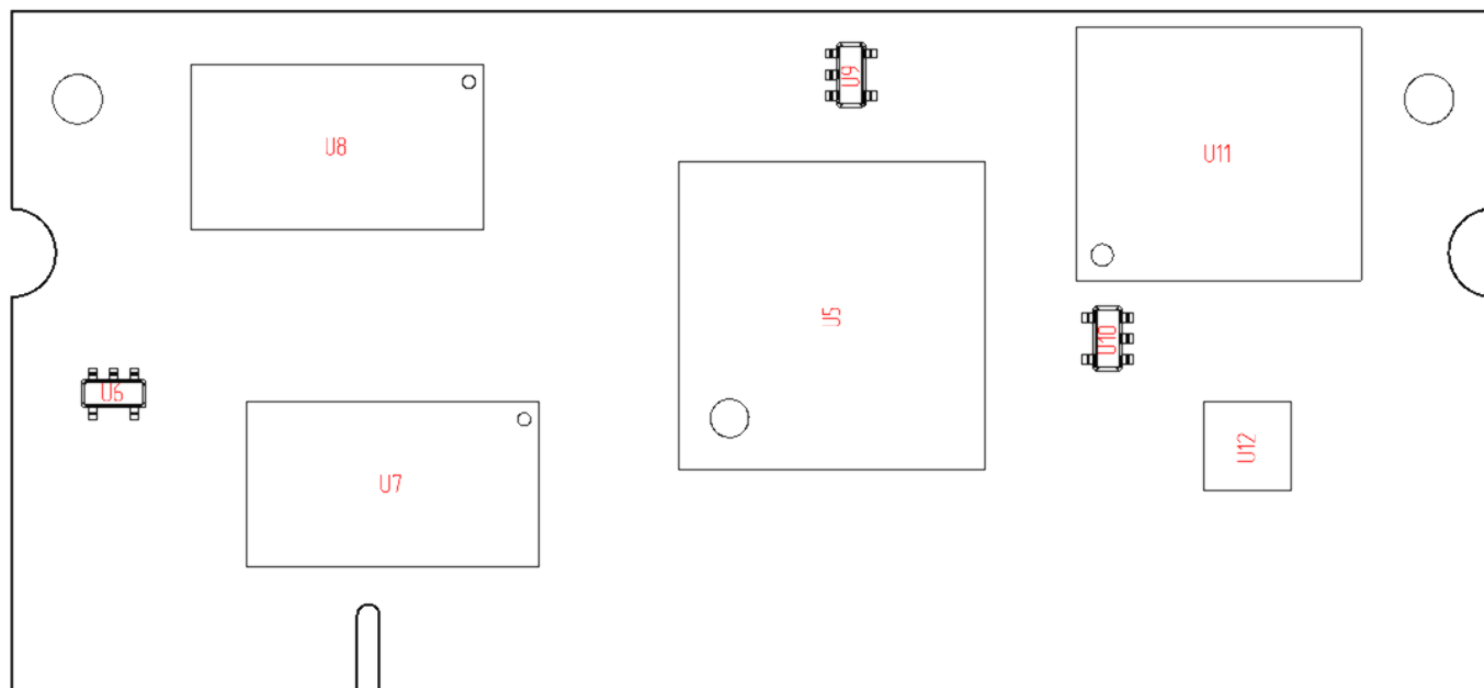
Рисунок 3: Расположение компонентов на плате. Вид сверху
